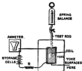
FIG. 4. S. P. Thompson's permeameter.
