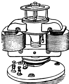
FIG. 10. Hysteresis Meter.
