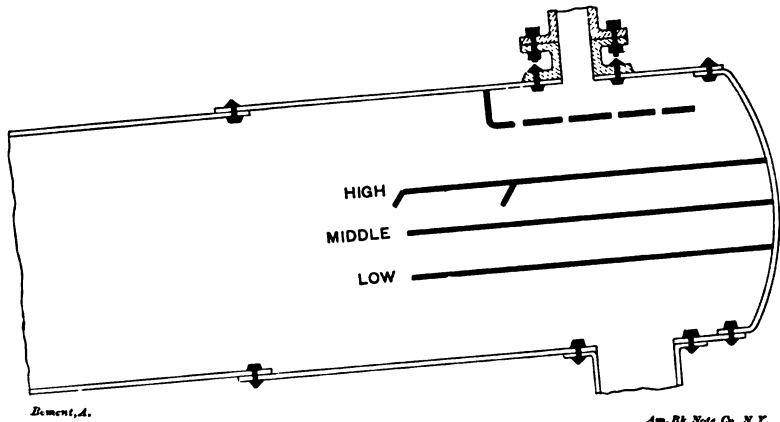
FIG. 95.—STYLE OF BAFFLES.
